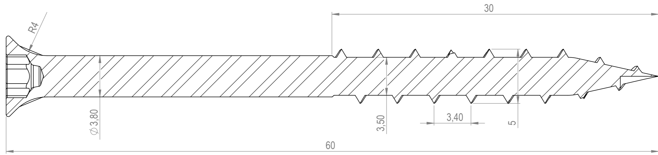
B-B (5 : 1)
